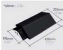
Q90 ATICA RIDGE 120°
