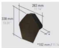
Q147 45° RIDGE END CAP
