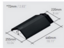
Q120 ANGULAR RIDGE
