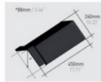
Q110 ATICA COLLAR RIDGE
