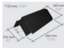
Q145 45° RIDGE
